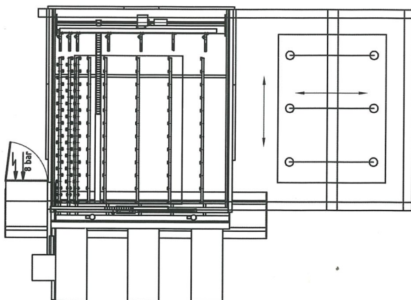
Euro 5.1 mit modular erweiterbarem Beschickungs- und Lagersystem
